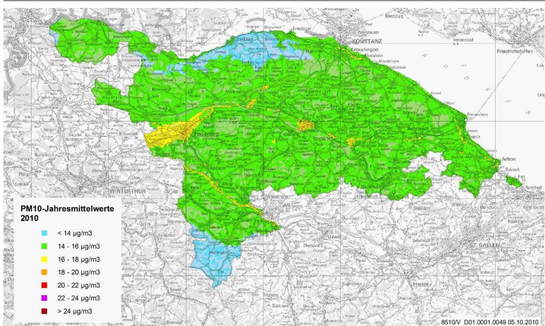
Abbildung 61: Prognose Feinstaubbelastung 2010
