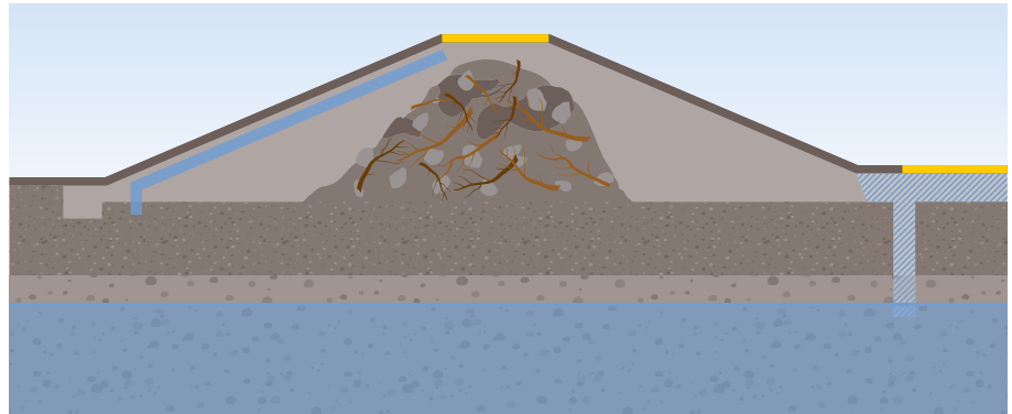
Die alten Dämme werden nach einheitlichen, zeitgemässen Standards saniert.
