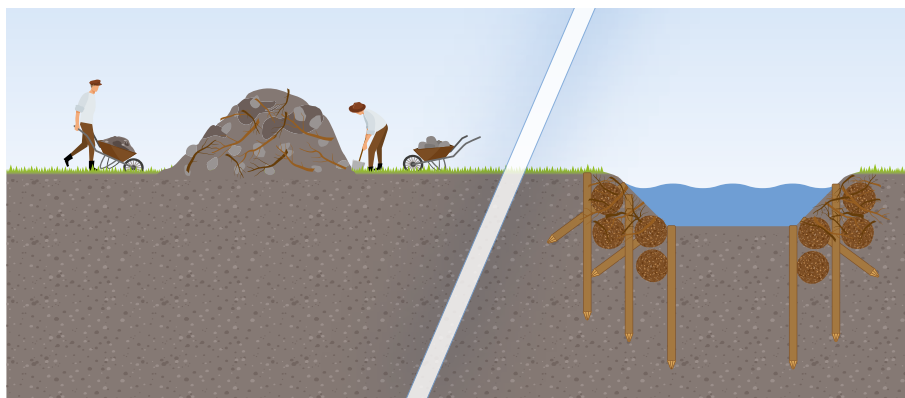
1870–1890: Für die Sicherung des Mittelgerinneufers wurden «Wuhren» verwendet, d. h. durch Pfahlreihen gestützte «Wuhrhäge», die aus biegsamem Holz, Buschwerk und Flechtwerk hergestellt wurden.
