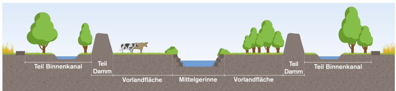
Ist-Zustand: Binnenkanäle, Damm, Vorland, verbautes Mittelgerinne
