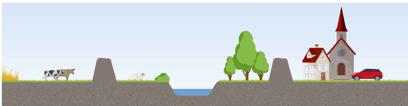
Das Schutzsystem der Thur (schematisch überzeichnet): Mittelgerinne, Thurvorland, Hochwasserdamm. Bei Niedrigwasser hat die Thur ausreichend Platz in ihrem Bett.
