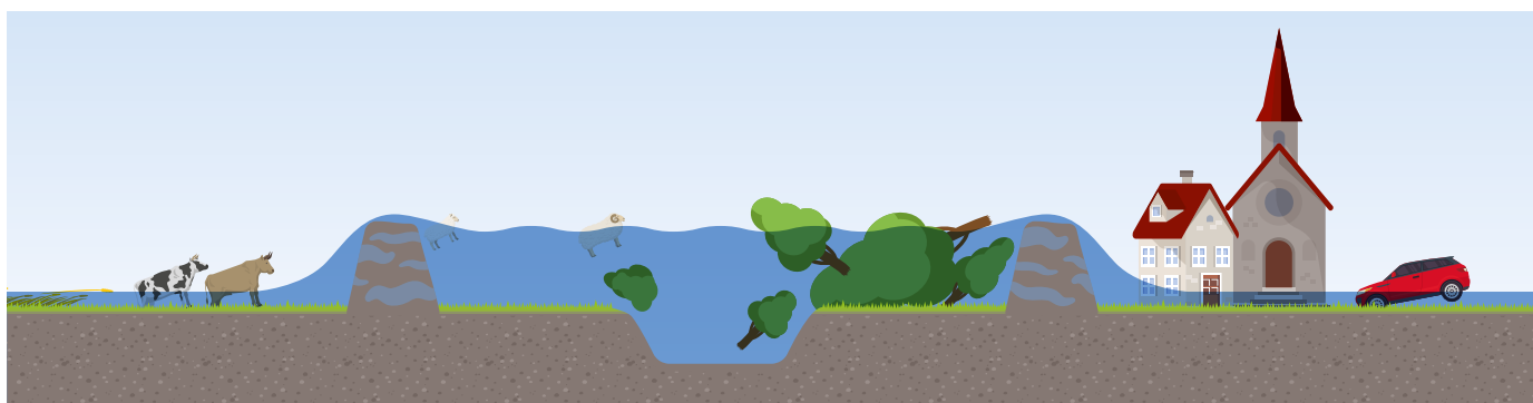
Mögliche Situation heute bei einem Hochwasser ab der Stärke HQ_{30} : Der Wasserabfluss zwischen den Dämmen ist nicht mehr gewährleistet. Die Dämme können brechen oder überspült werden.
