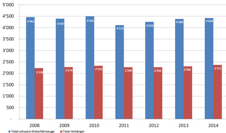
Bestandesentwicklung der Fahrzeuge > 3.5 t
